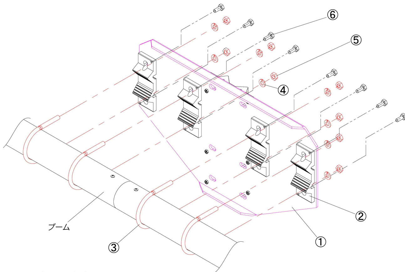
図17: ブーム側の組立図
