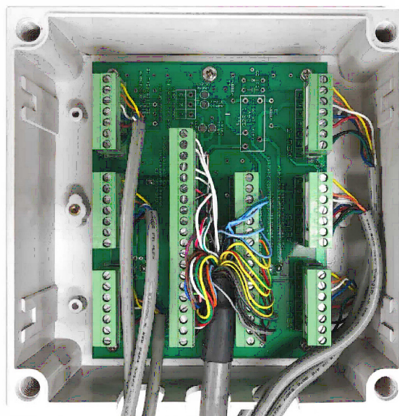
図16: 6エレメントモデルのジャンクションボックス内部
