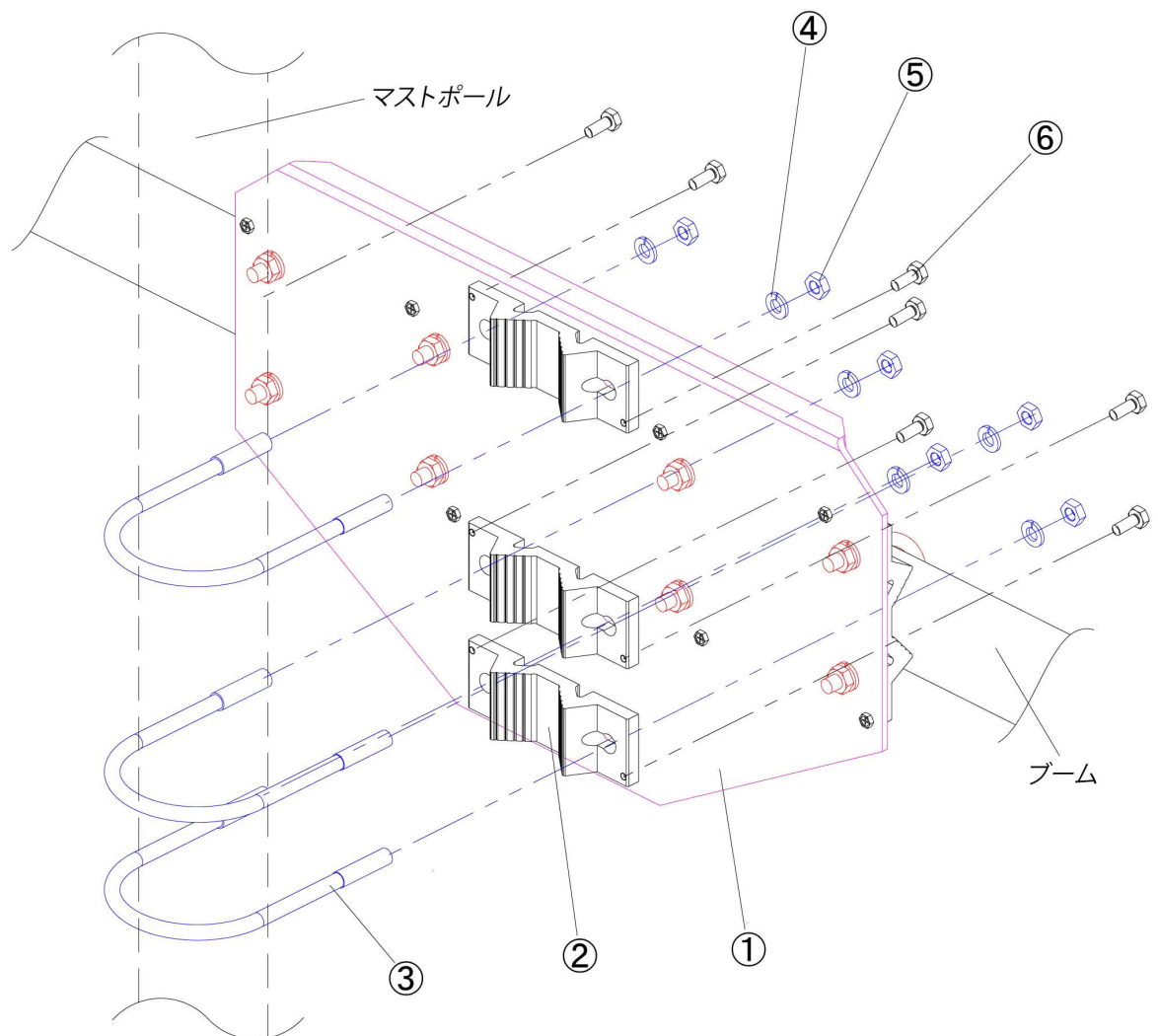
図18: マストポール側の組立図
