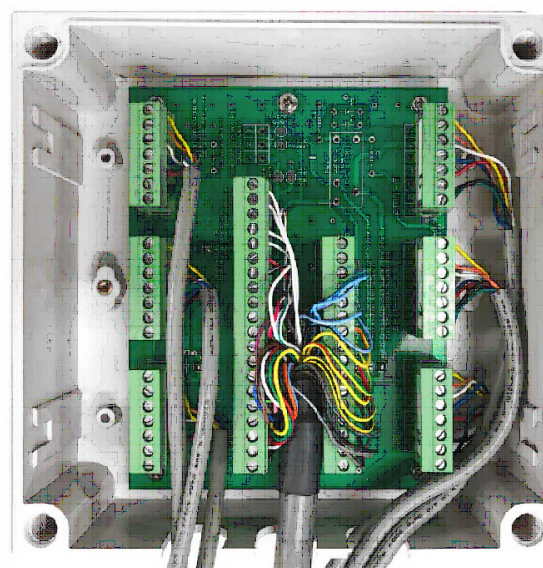
図11：6エレメントモデルのジャンクションBOX内部
