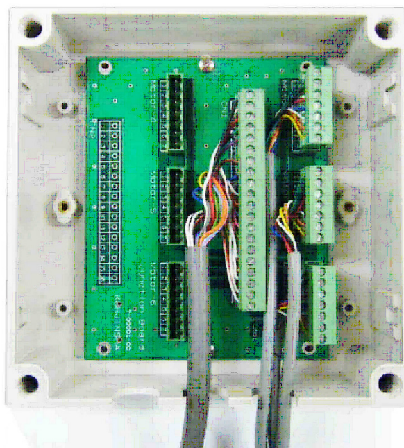
図14: 3 Elementモデルのジャンクションボックス内部です
