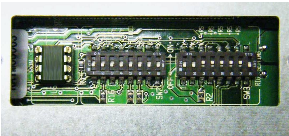
図40：上記の写真を参考にディップスイッチ（白い突起部分）を上下に動かして設定を行ってください。
