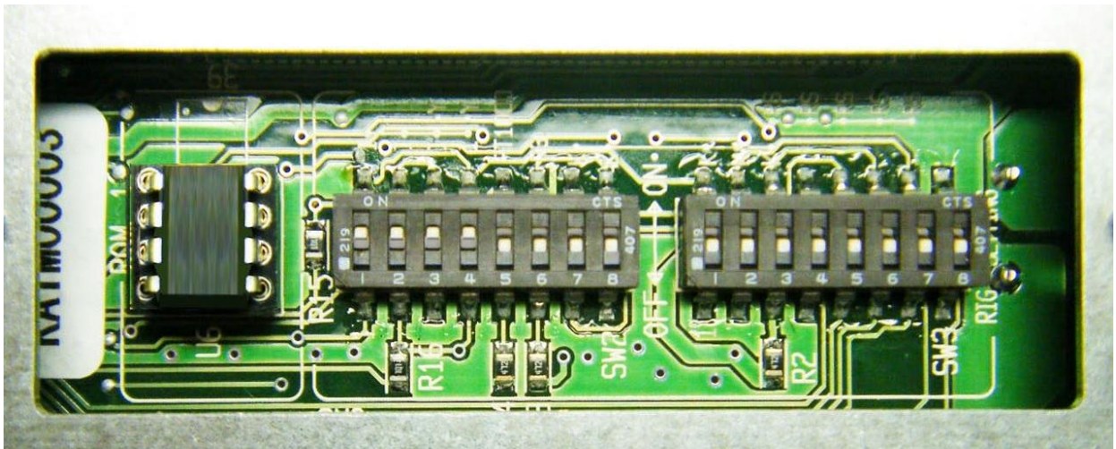
図41：上記の写真を参考にディップスイッチ（白い突起部分）を上下に動かして設定を行ってください。
